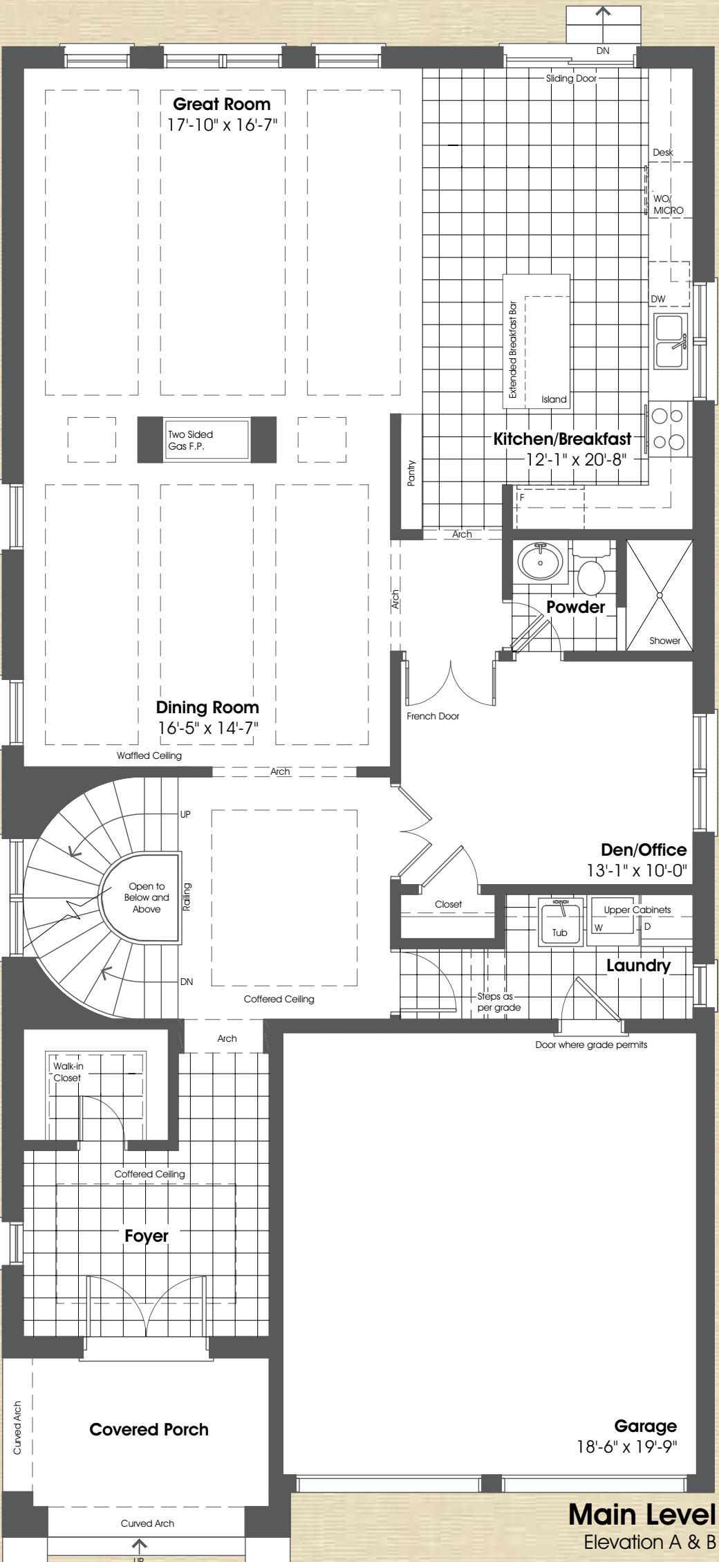
ELEV.A
